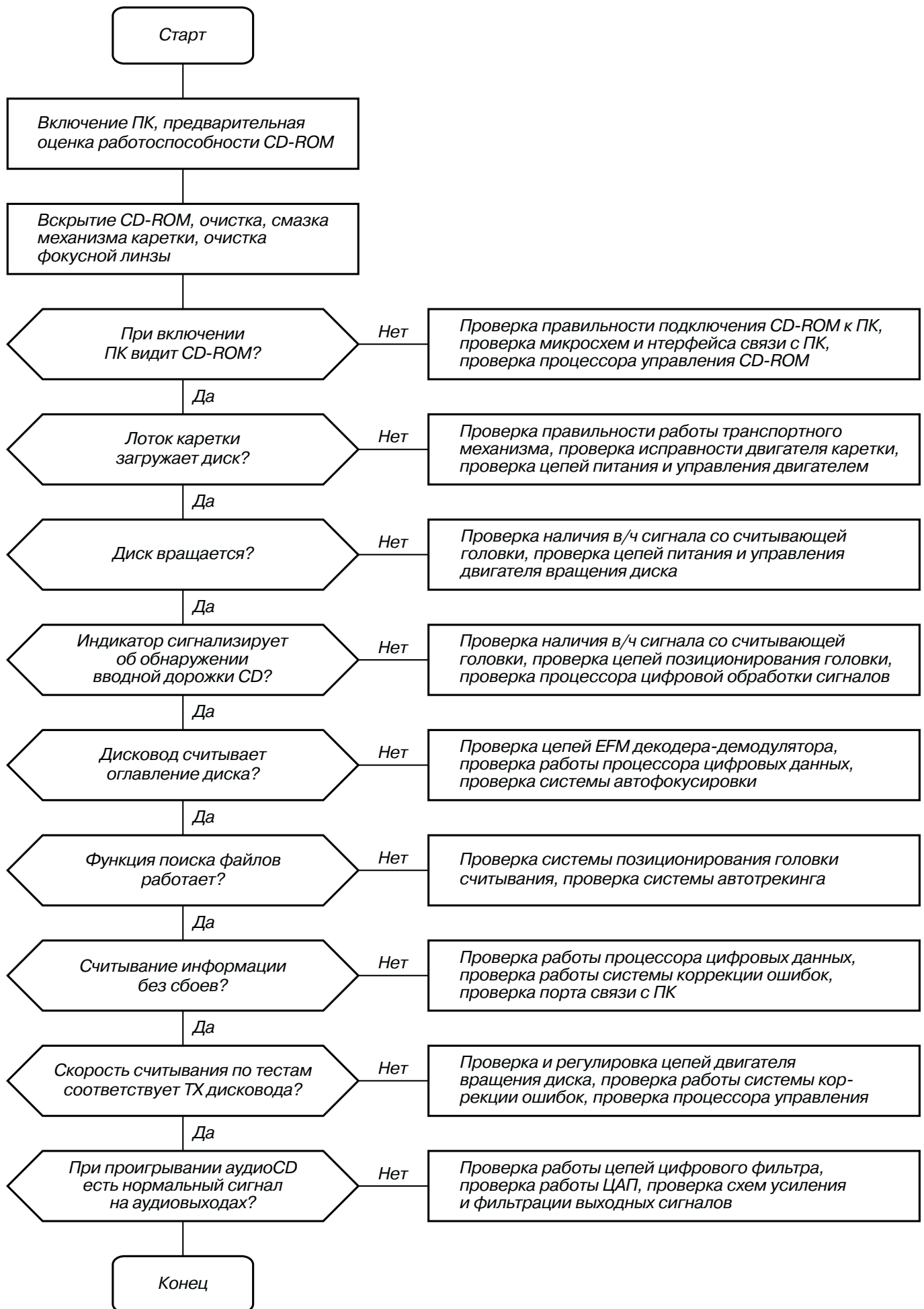
Рис. 7. Алгоритм поиска неисправностей CD-ROM
