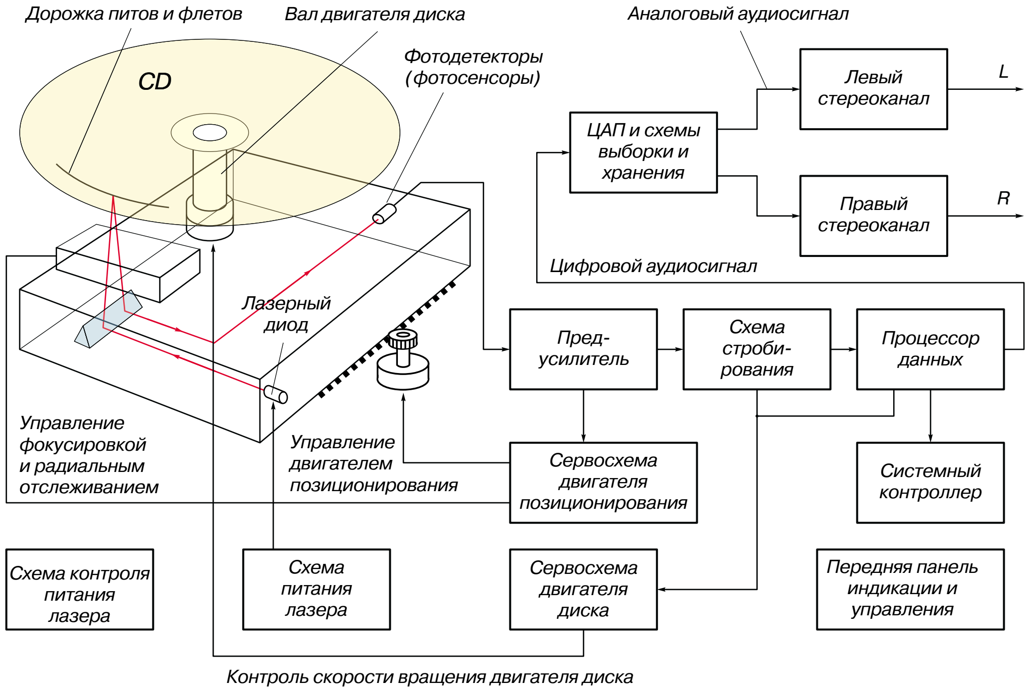
Рис. 1. Структурная схема CD-ROM
