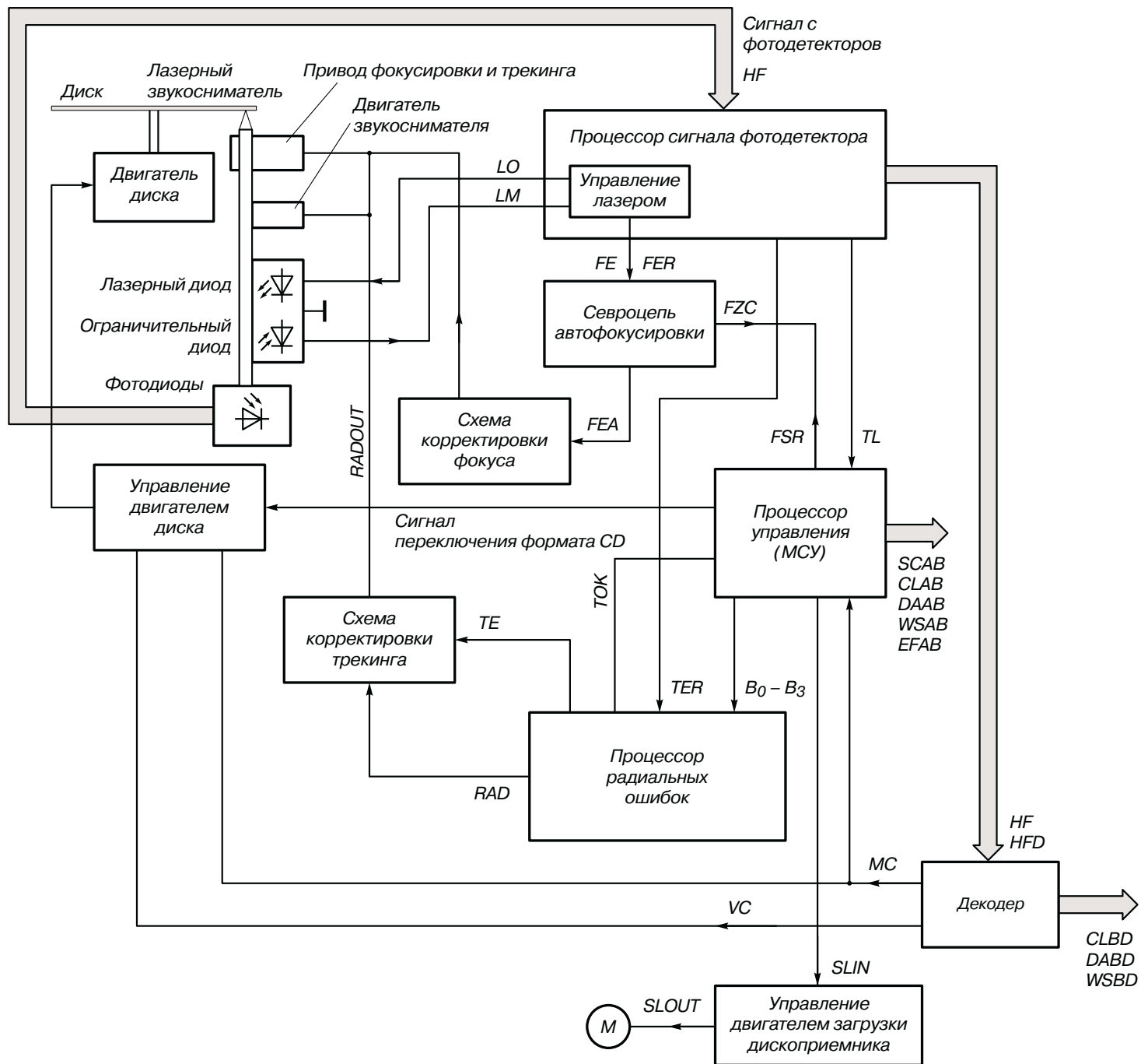
Рис. 3. Структура связей оптико-электронной системы считывания информации
